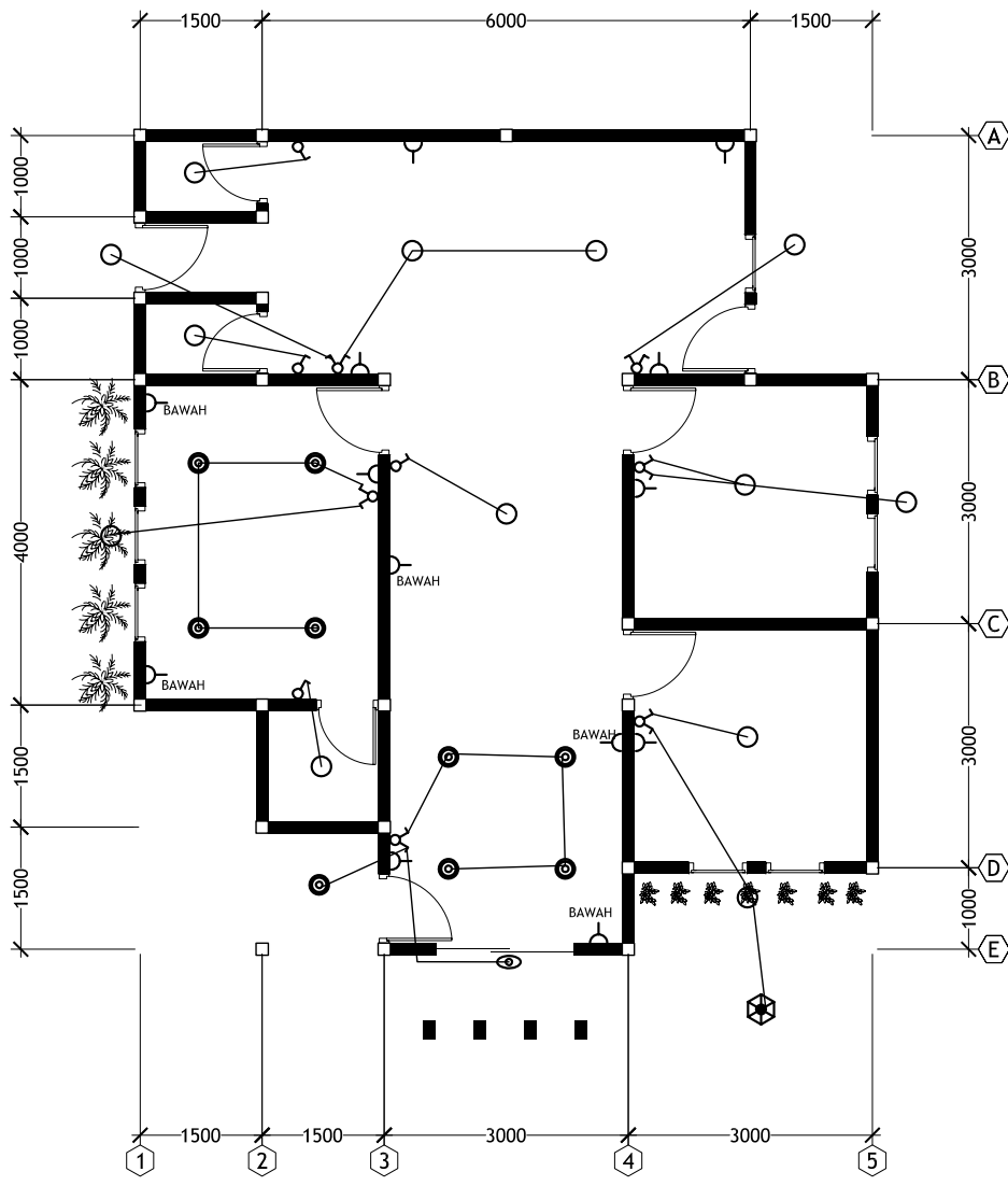
DENAH ELEKTRIKAL SKALA 1:100
