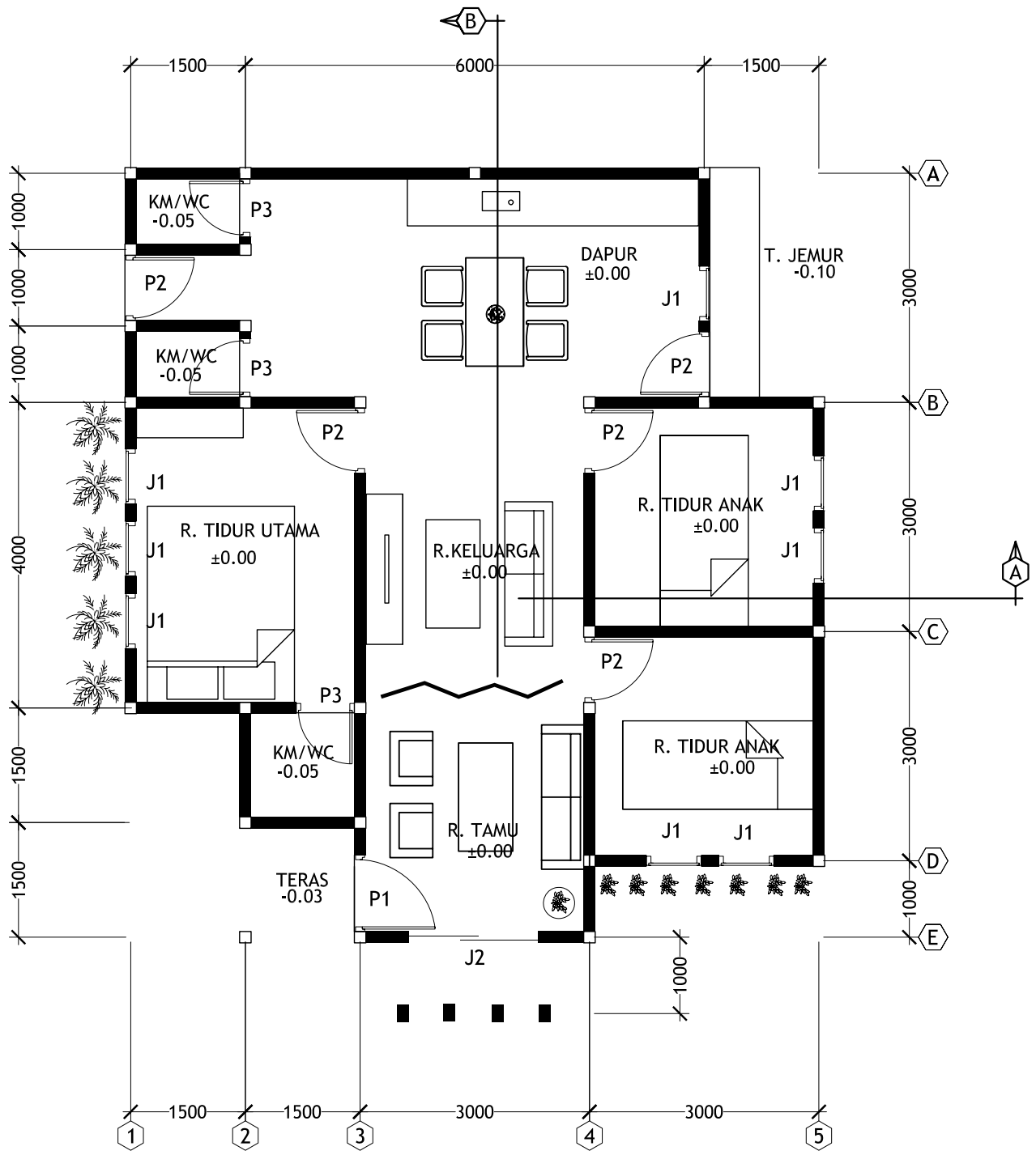
DENAH RENCANA SKALA 1:100
