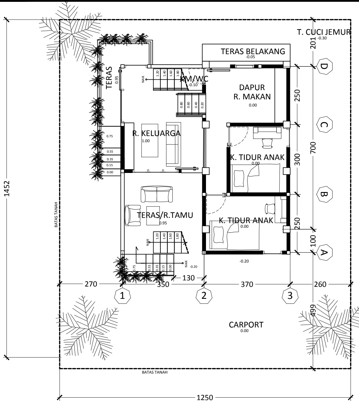
DENAH LT. 1 SKALA 1:125
