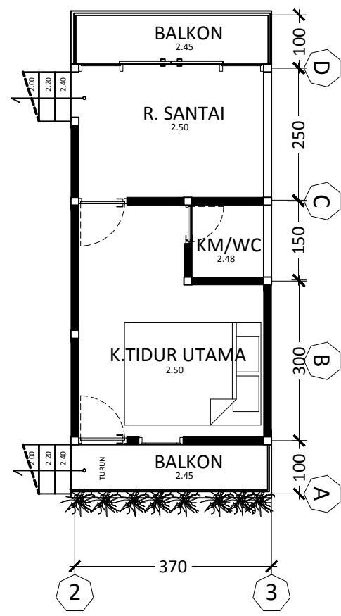
DENAH LT. 2 SKALA 1:125
