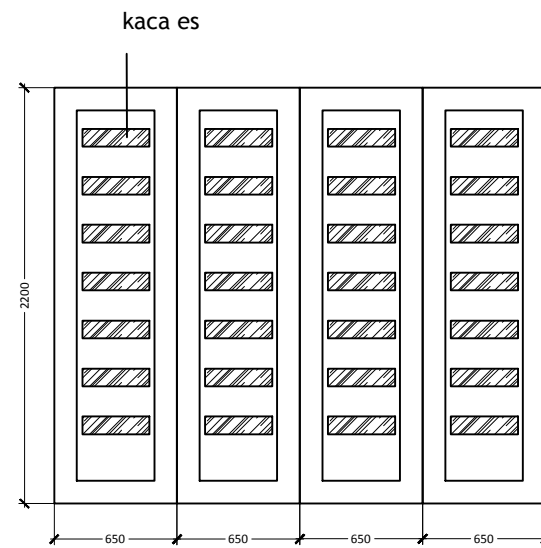
PINTU GARASI LIPAT, P4
