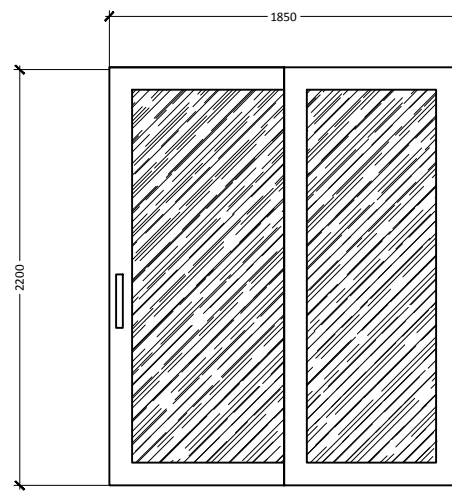
RENCANA PJ1 SLIDING
