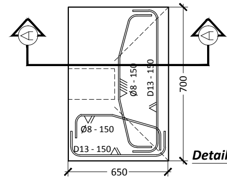
Detail Pondasi F-1
