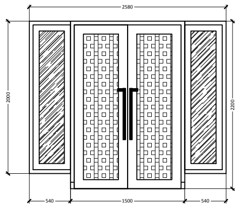
PINTU RUANG TAMU
