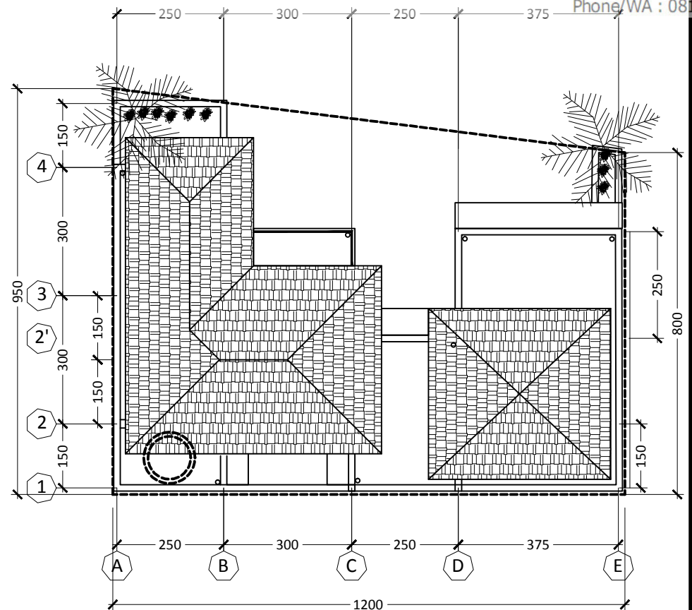
RENCANA ATAP SKALA 1:125
