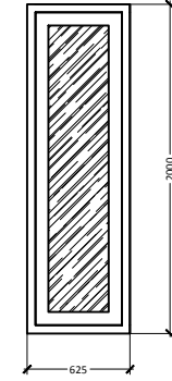
JENDELA KAMAR BELAKANG
