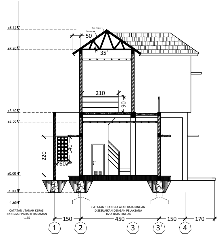
POTONGAN B SKALA 1:125
