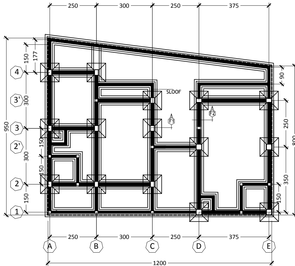
DENAH PONDASI SKALA 1:125
